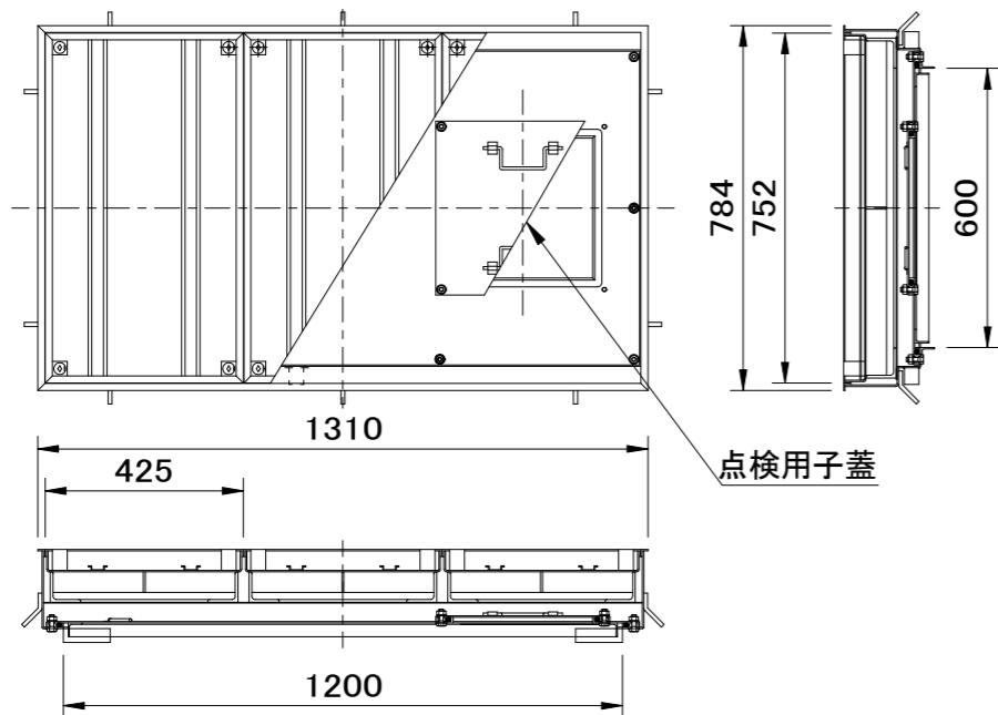
点検口用子蓋付 SF-60×120BMP-6 特
