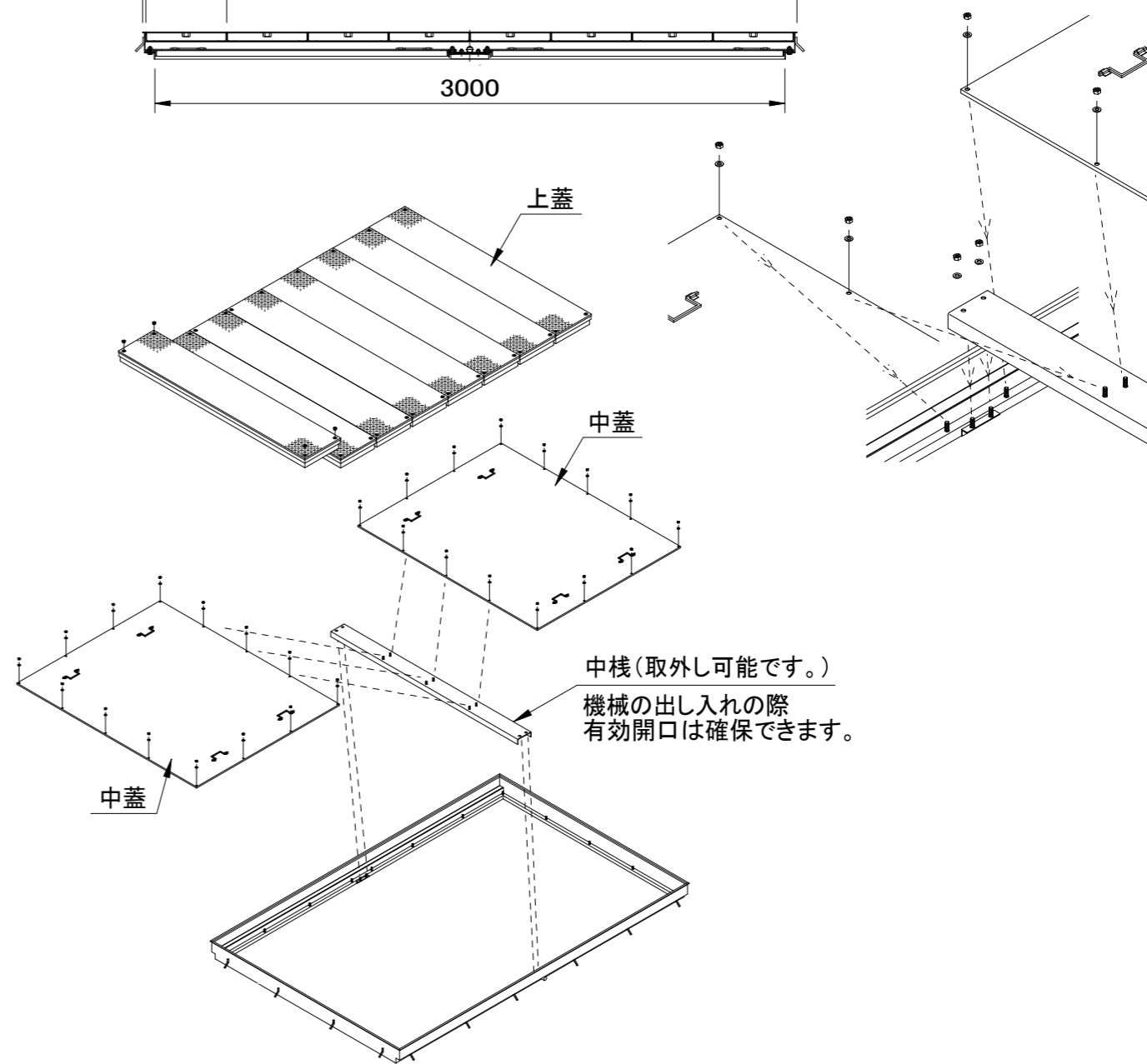
中蓋2分割（簡易防水防臭型） SF-150×300CMP-1 特
