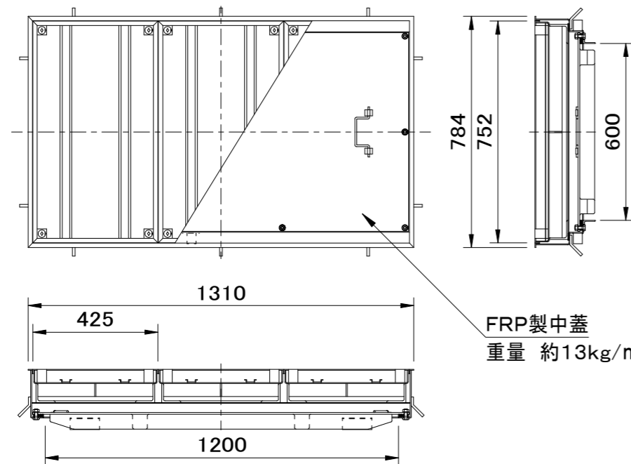
中蓋FRP製 SF-60×120BMP-6 特
