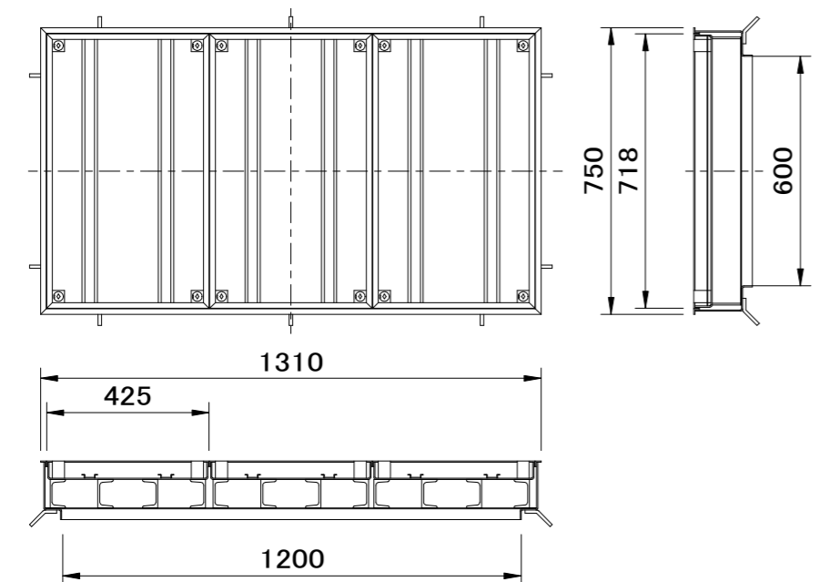
適応荷重 T-14 SF-60×120BM-14
