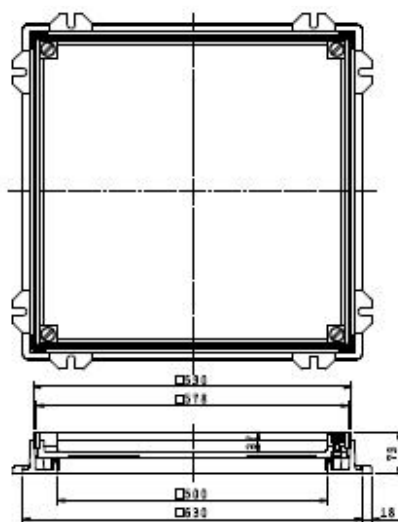
SF-50CT-8型 製品図
