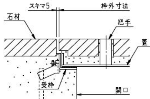
仕上げ後に目地が見えない タイプの化粧蓋(断面図)
