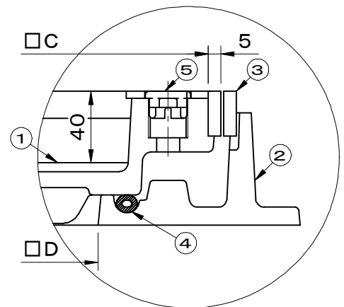
把手部拡大図
