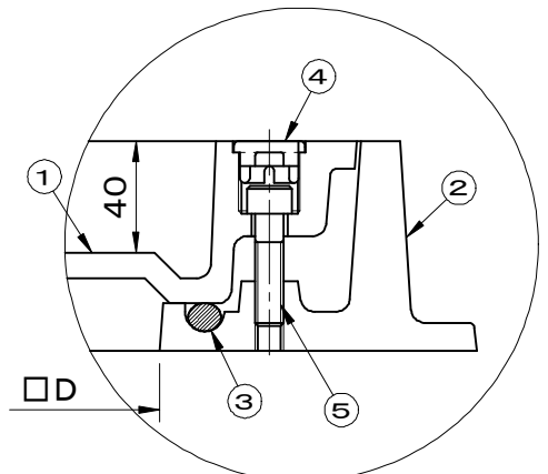
ボルト固定部拡大図
