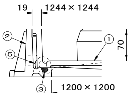
拡大図
