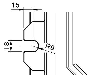
アンカー切欠き寸法
