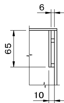
把手穴部平面寸法
