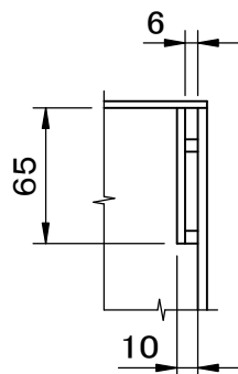
把手穴部平面寸法
