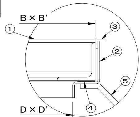
拡大図
