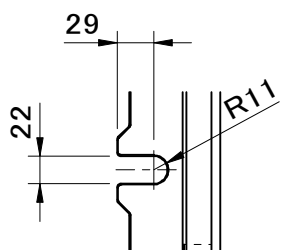
アンカー切欠き寸法
