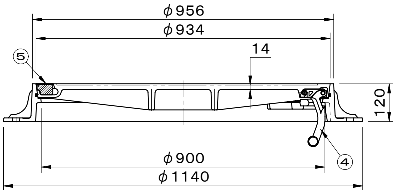
A断面図
