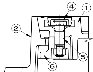
施錠部詳細図
