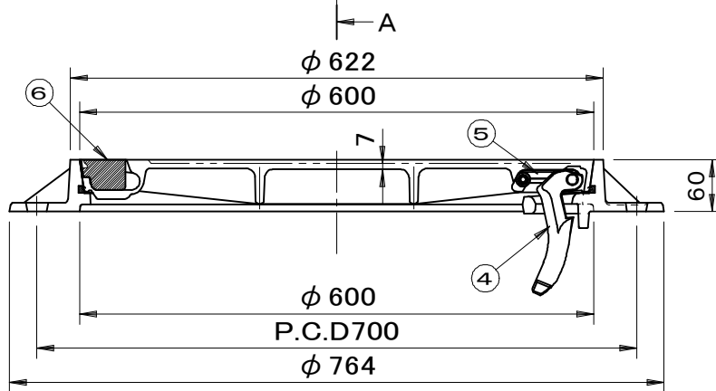
A断面図
