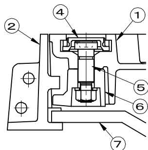
施錠部詳細図
