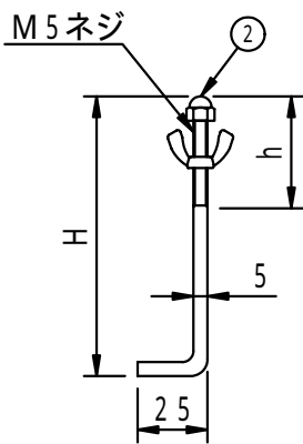
取付金具
