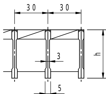
メインバー断面詳細図 h = 44 の場合
