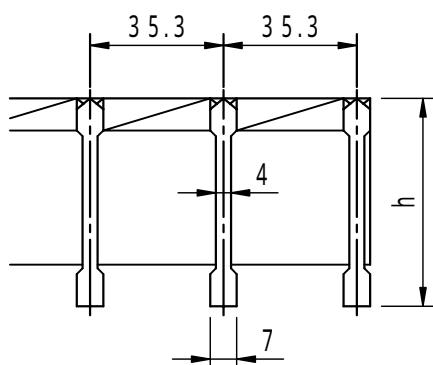
メインバー断面詳細図 h = 55, 65 の場合
