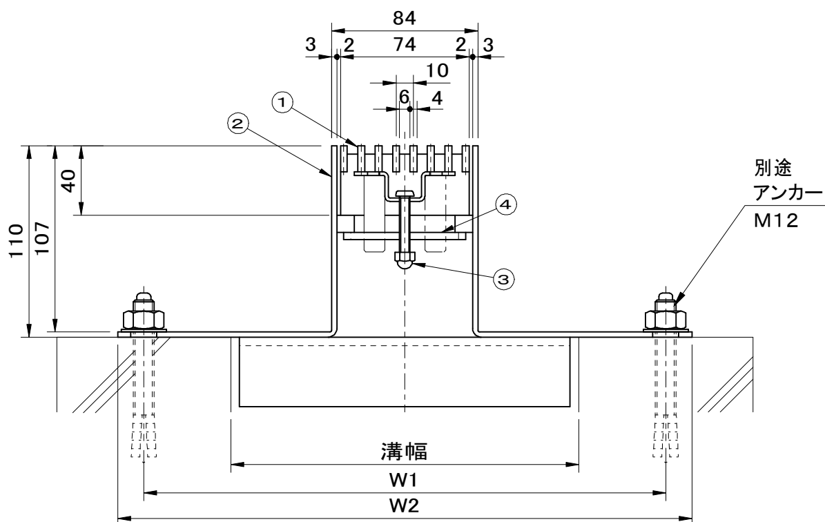
断面拡大図
