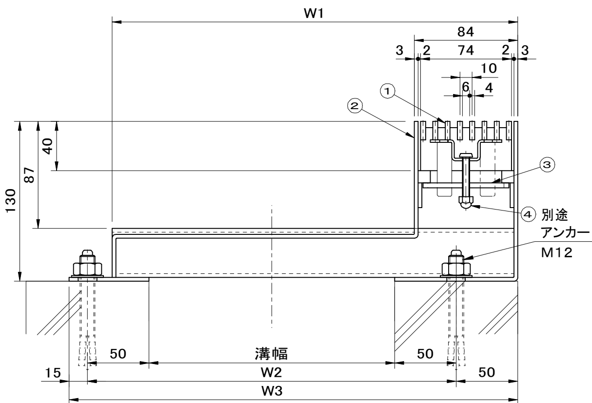
断面拡大図
