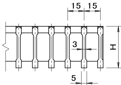
メインバー断面詳細図
