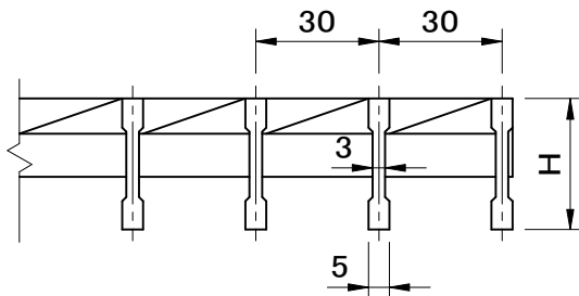
メンバー断面詳細図
