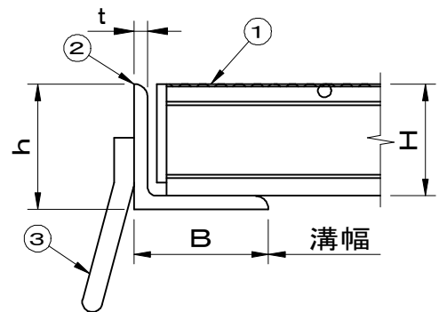
拡大図
