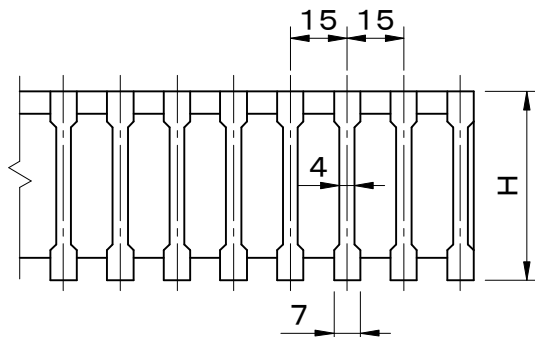
メンバー断面詳細図
