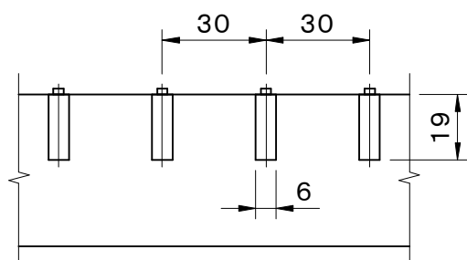
メインバー断面詳細図
