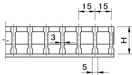
メインバー断面詳細図
