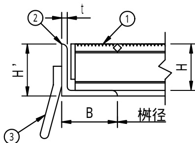
拡大図
