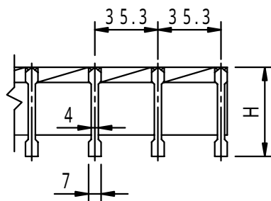
メンバー断面詳細図
