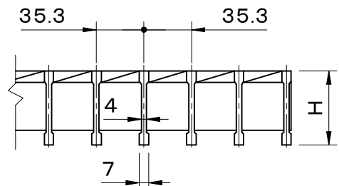
メインバー断面詳細図
