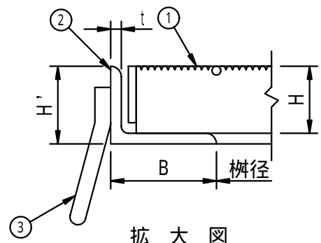
メインバー上部拡大図
