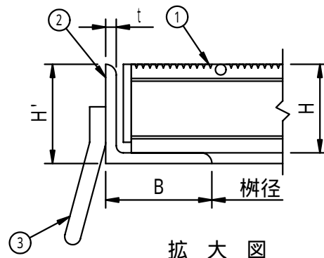
メインバー上部拡大図
