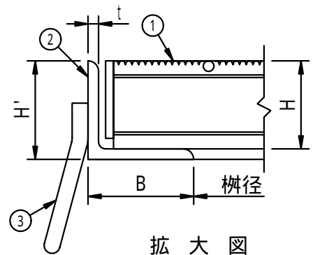
メインバー上部拡大図
