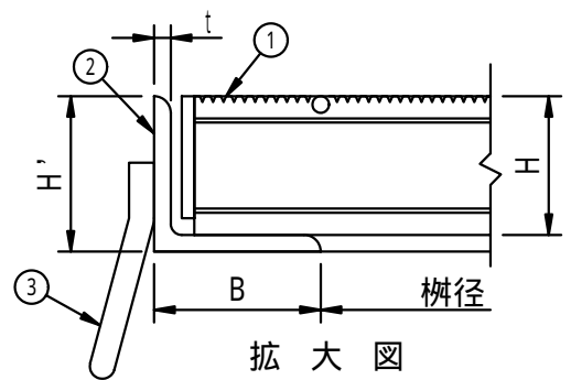
メインバー上部拡大図
