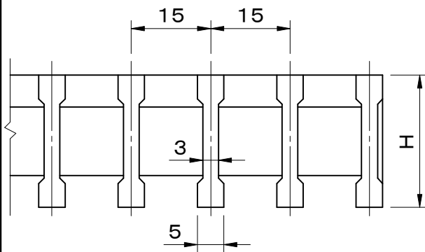
メインバー断面詳細図
