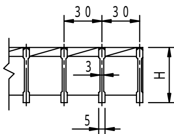
メンバー断面詳細図
