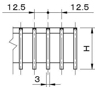
メインバー断面詳細図
