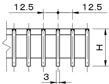
メインバー断面詳細図
