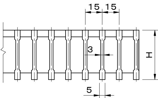
メンバー断面詳細図
