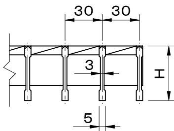
メインバー断面詳細図
