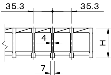
メインバー断面詳細図
