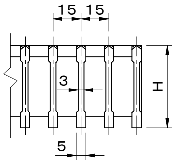
メインバー断面詳細図
