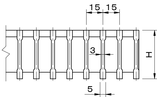
メインバー断面詳細図
