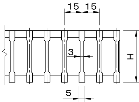
メインバー断面詳細図
