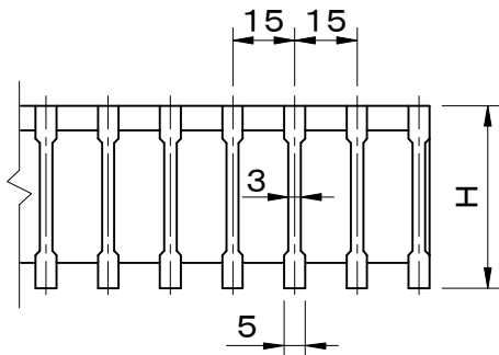
メインバー断面詳細図
