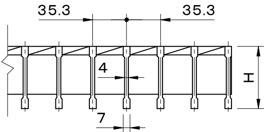
メインバー断面詳細図
