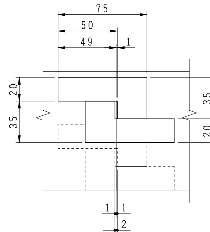
連結ジョイント部分
