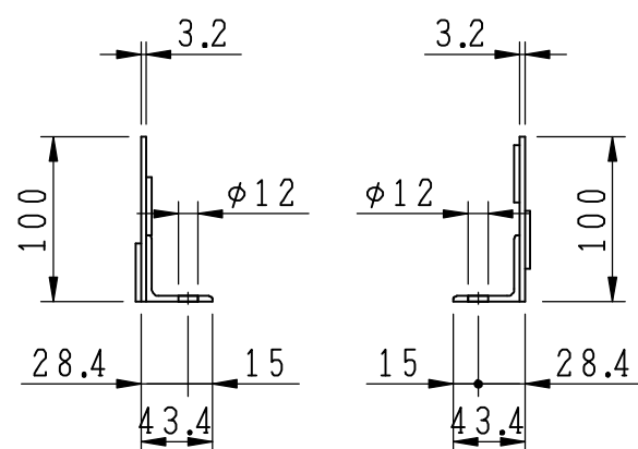
A 矢視図
