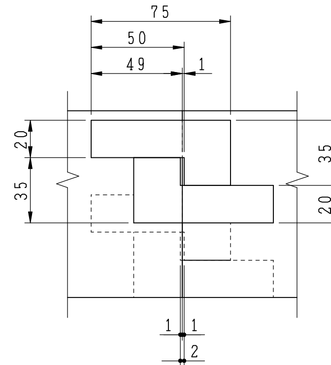
連結ジョイント部分
