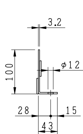
A 矢視図
